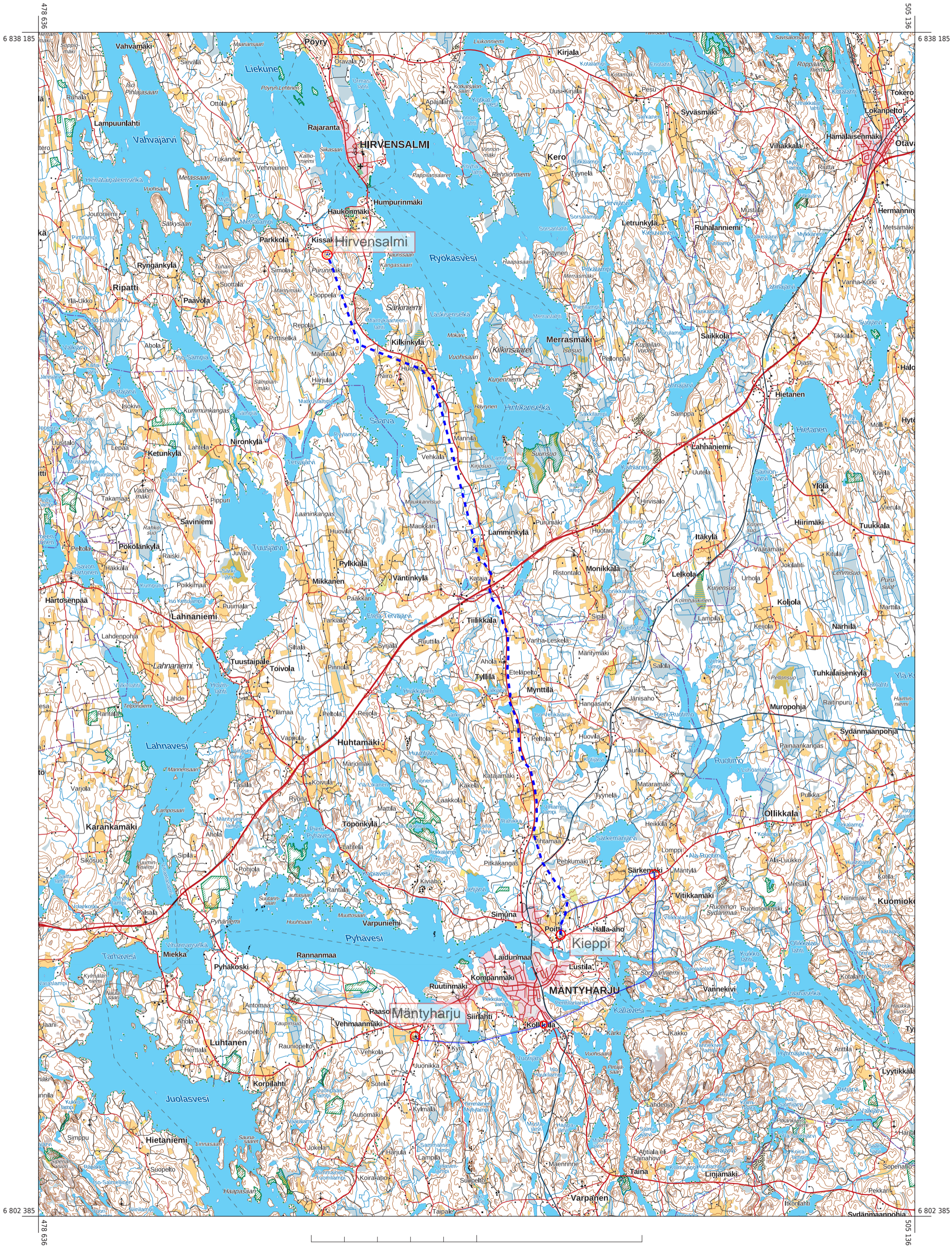
0 5 Suunniteltu 110 kV Kieppi-Hirvensalmi
